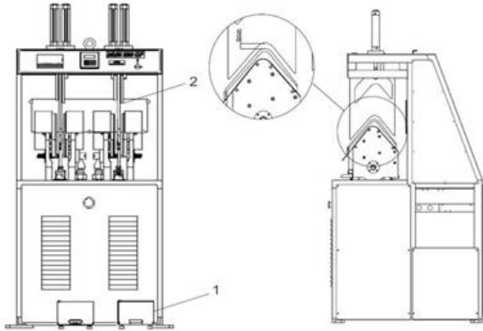
Figura 8: Máquina de cambrê facção - Vista frontal
